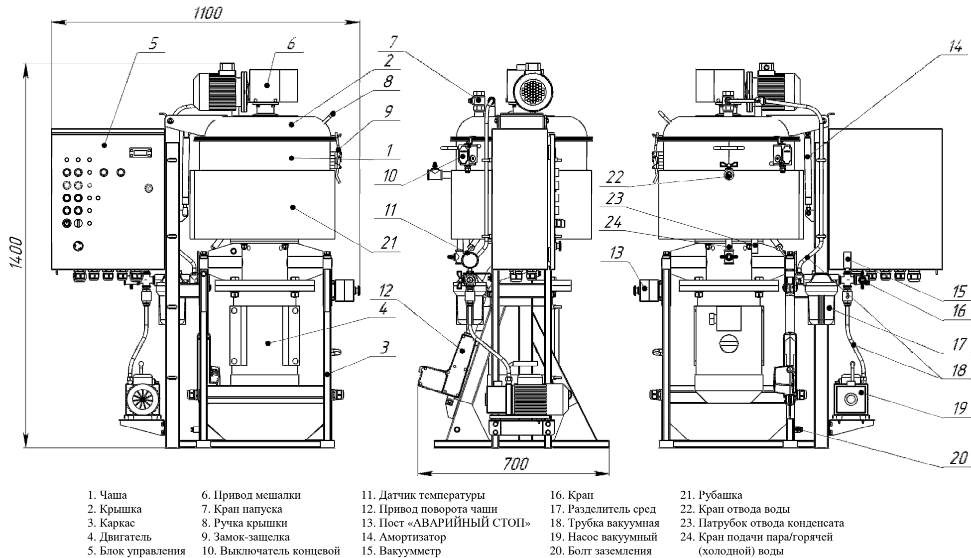
Рисунок 2. Куттер ИПКС-032-50П(Н); ИПКС-032-50РП(Н)
