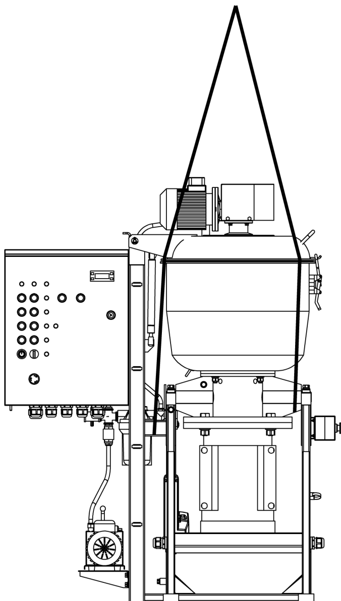
Рисунок 10. Схема строповки
