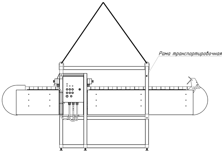
Рисунок 5. Устройство нарезки ИПКС-074-200МЧ(Н). Схема строповки
