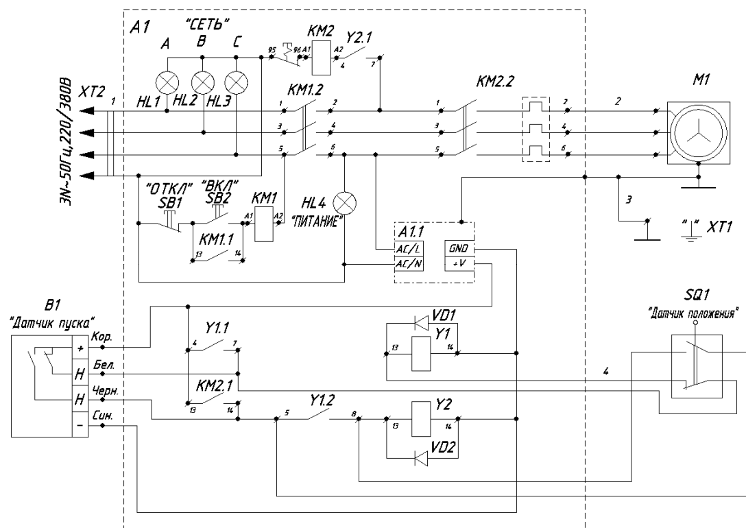
Рисунок 3. Машина укупорочная (маркировка крышек) ИПКС-127М
