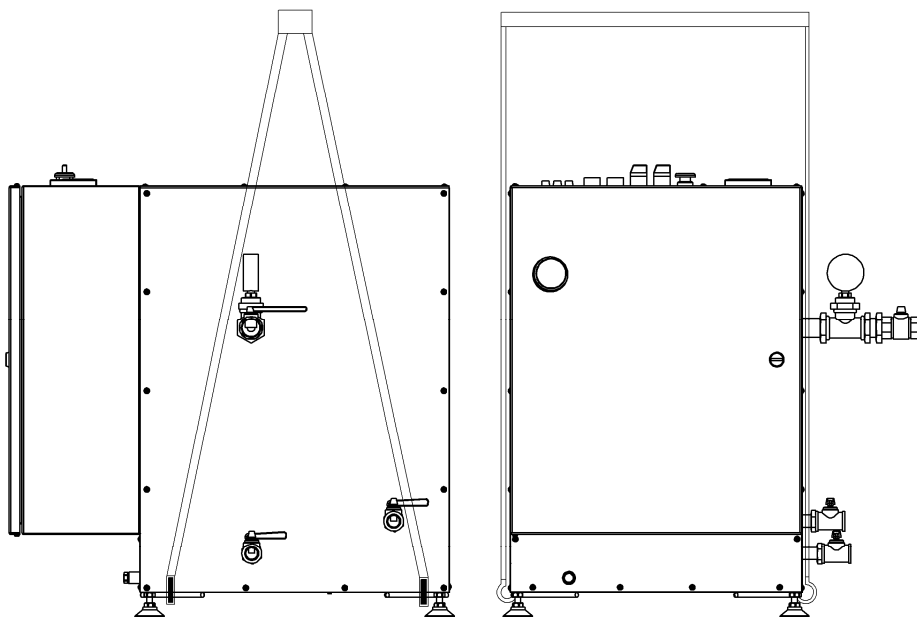
Рисунок 4. Парогенератор (регулируемый) ИПКС-129-100Р. Схема стропповки.
